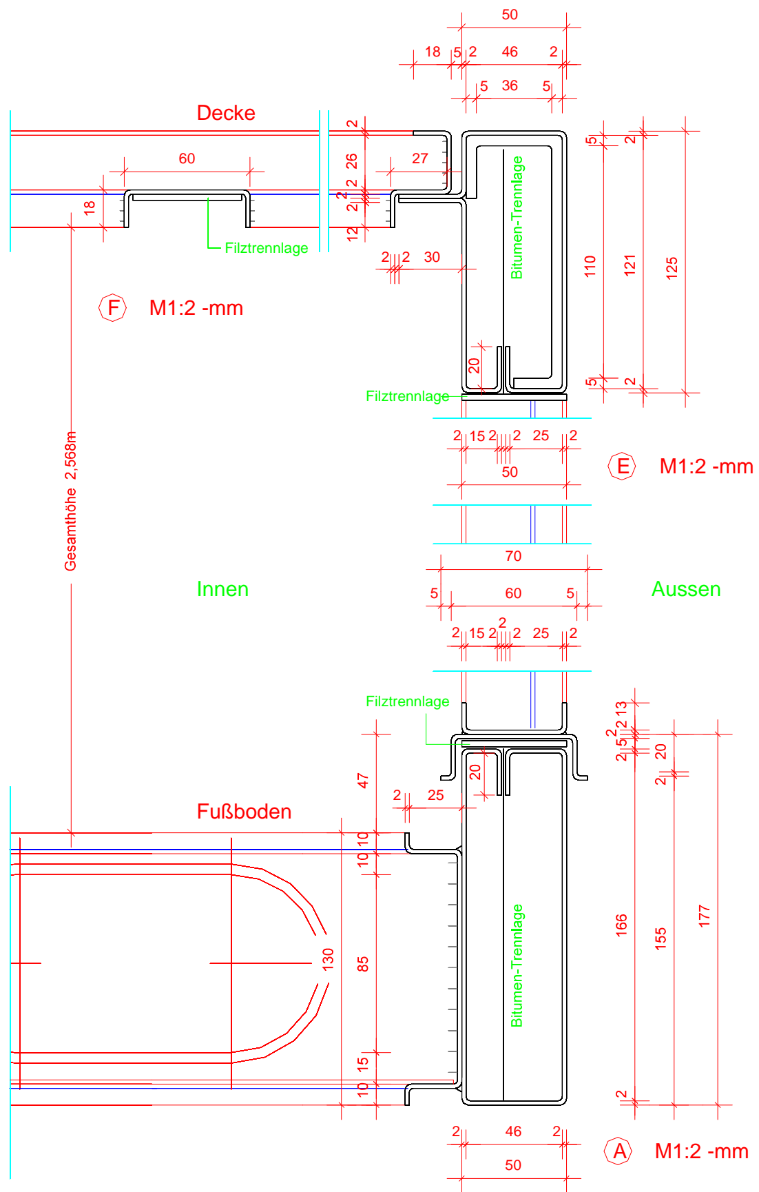
Vertikalschnitt Fassade C-C M1:2 -mm
