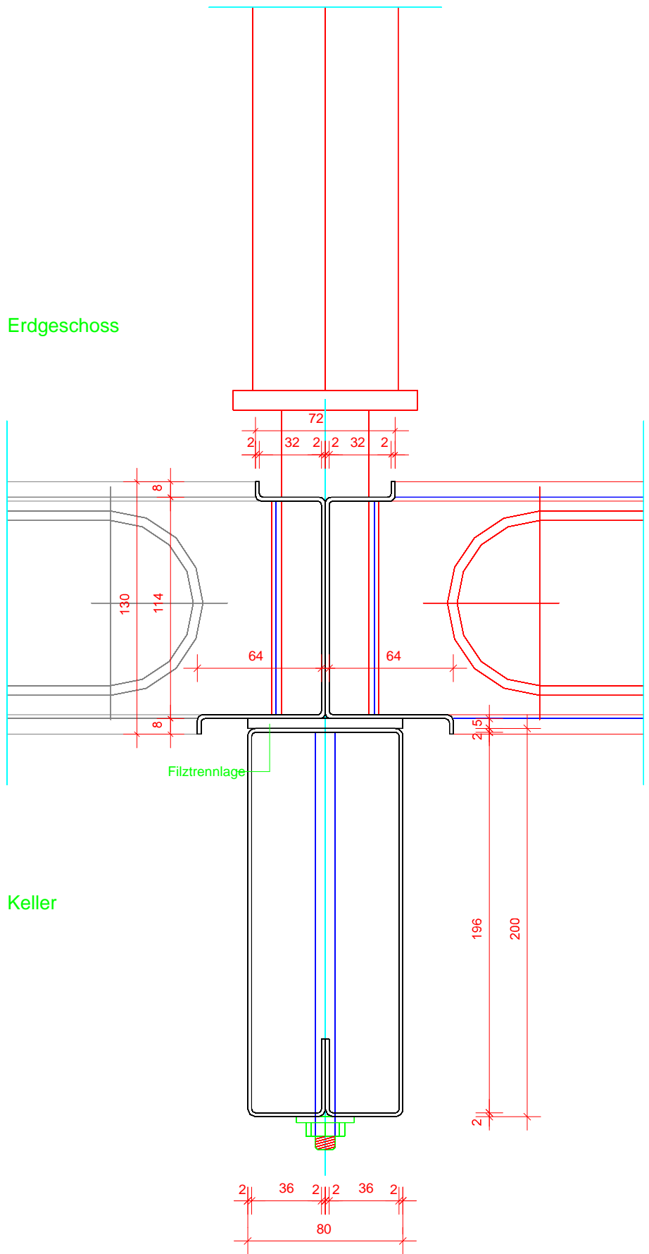
Portalrahmen / Unterzug, Detail 1 M1:2 -mm
